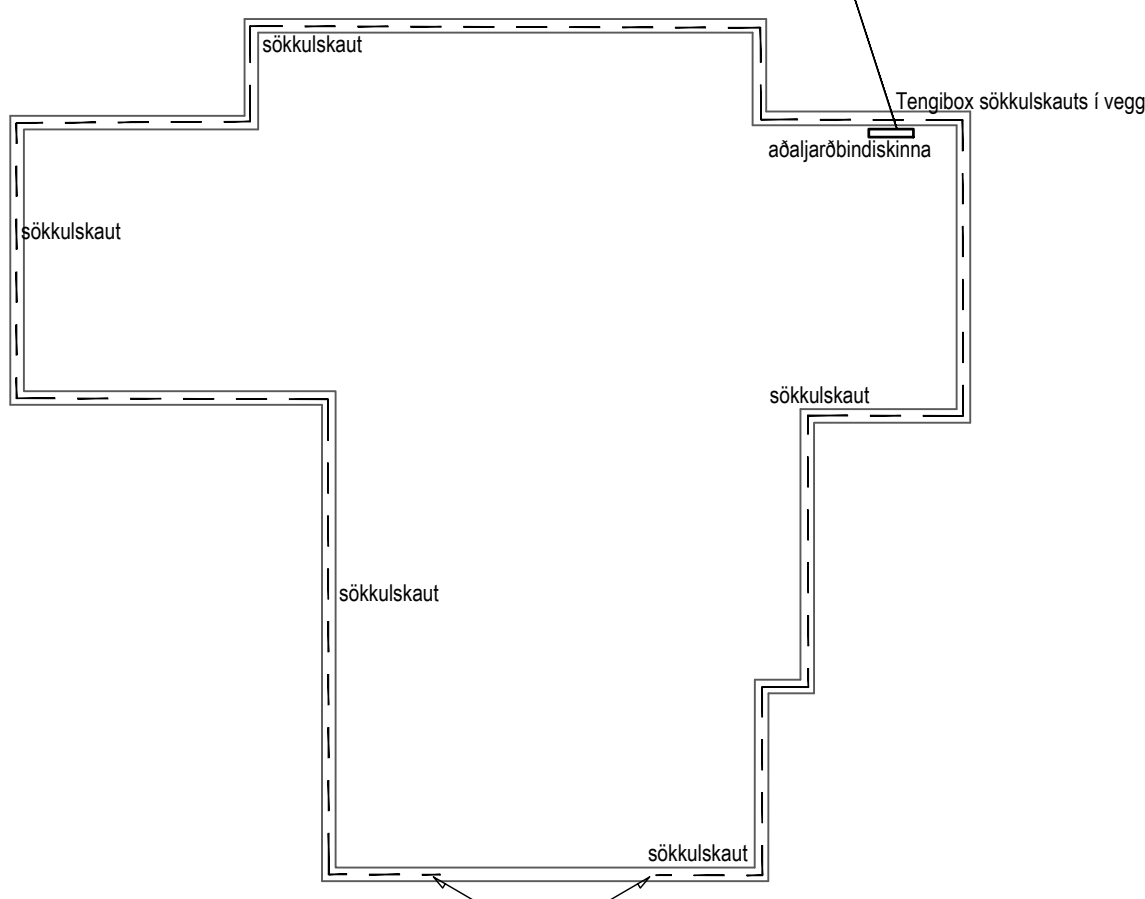
Jarðskaut og jarðtenging sökkulskauts 1:100
